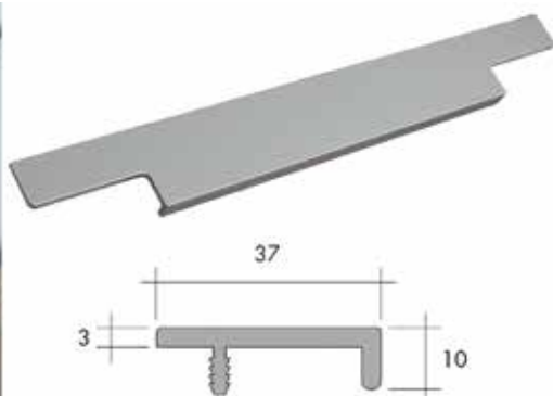
Poignée profil type 901.365
