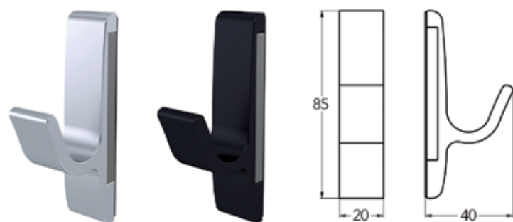
Crochet magnétique type 0150
