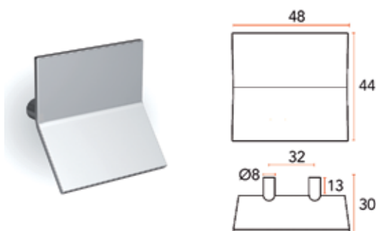
Bouton en zamac type 3405
