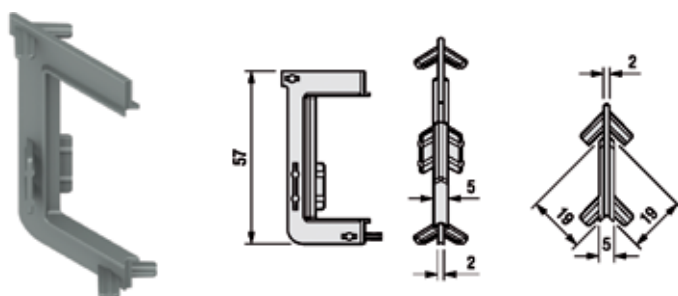
Pièce d'angle intérieure Gola L Led
