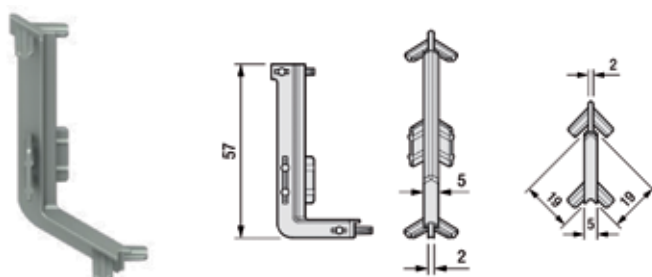
Pièce d'angle intérieure Gola L
