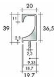
Profil poignée type 900303
