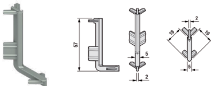
Pièce d'angle extérieure Gola L
