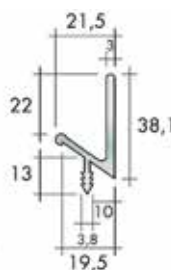
Profil poignée type 901.189
