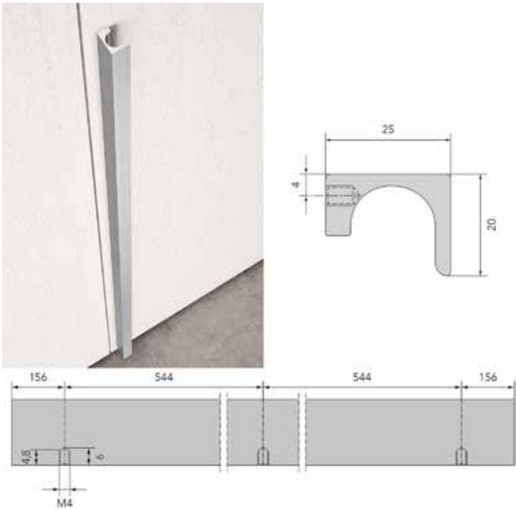
Poignée longue type 3610 - fixation: 3 x M4
