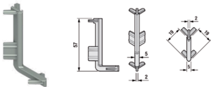
Pièce d'angle extérieure Gola L Led
