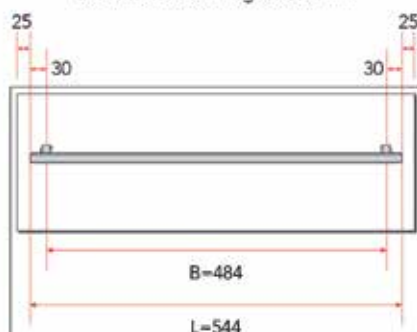
ex. armoire avec largeur 600 mm
